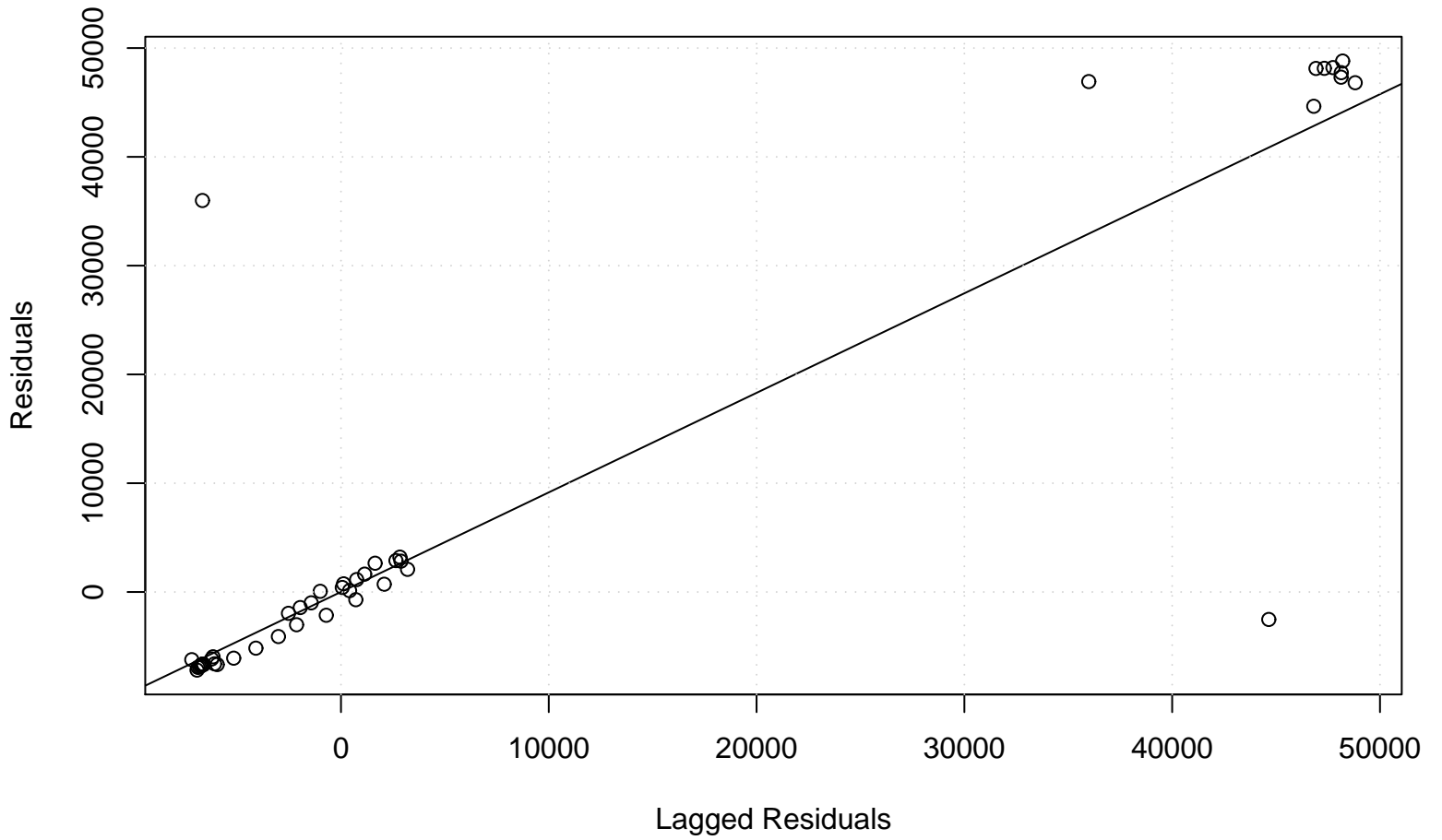
Lag plot
