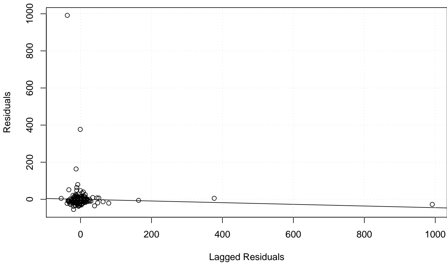
Lag plot
