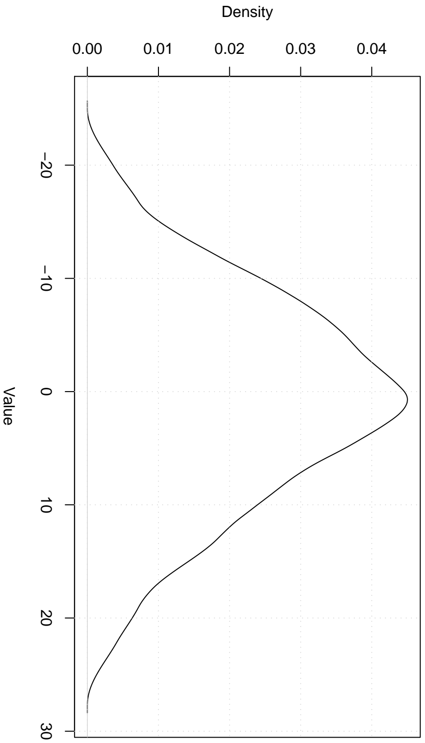
Cosine Kernel
