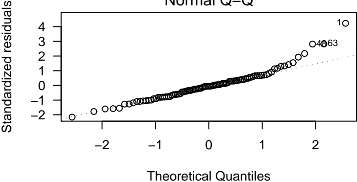
Normal Q-Q
