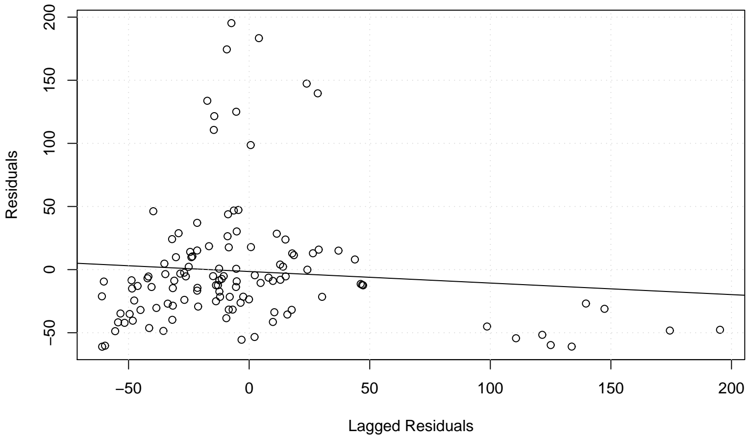
Lag plot
