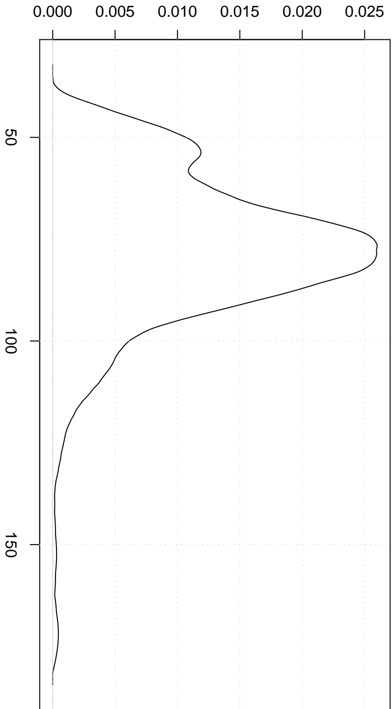
Optcosine Kernel
