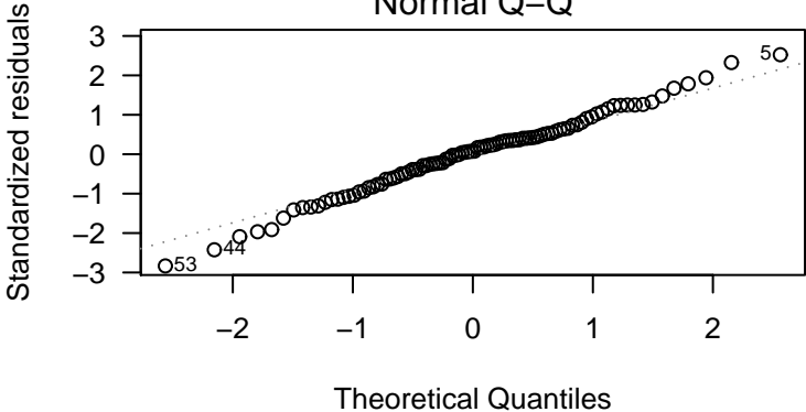
Normal Q-Q
