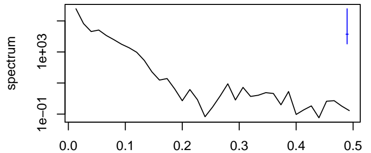
Trend
