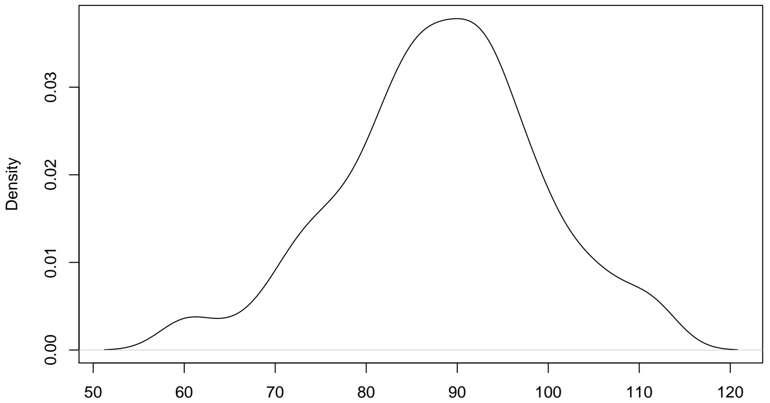
density.default(x = x)
