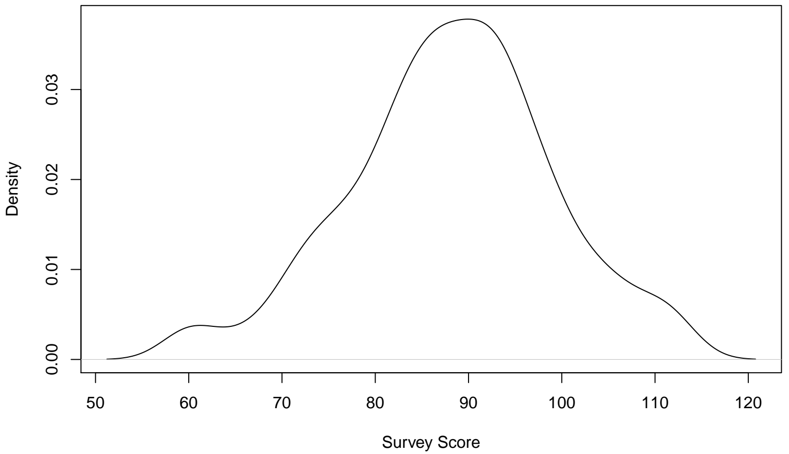
density.default(x = x)
