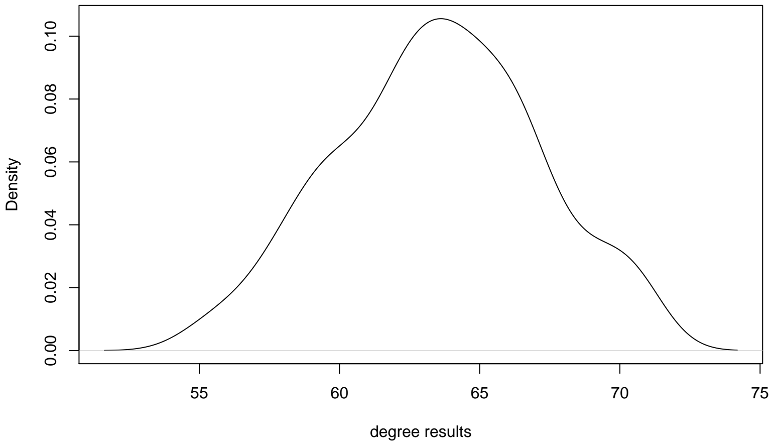
density.default(x = x)
