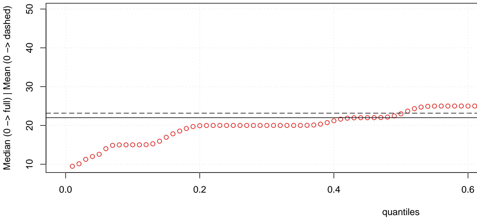
Harrell–Davis Quantiles
