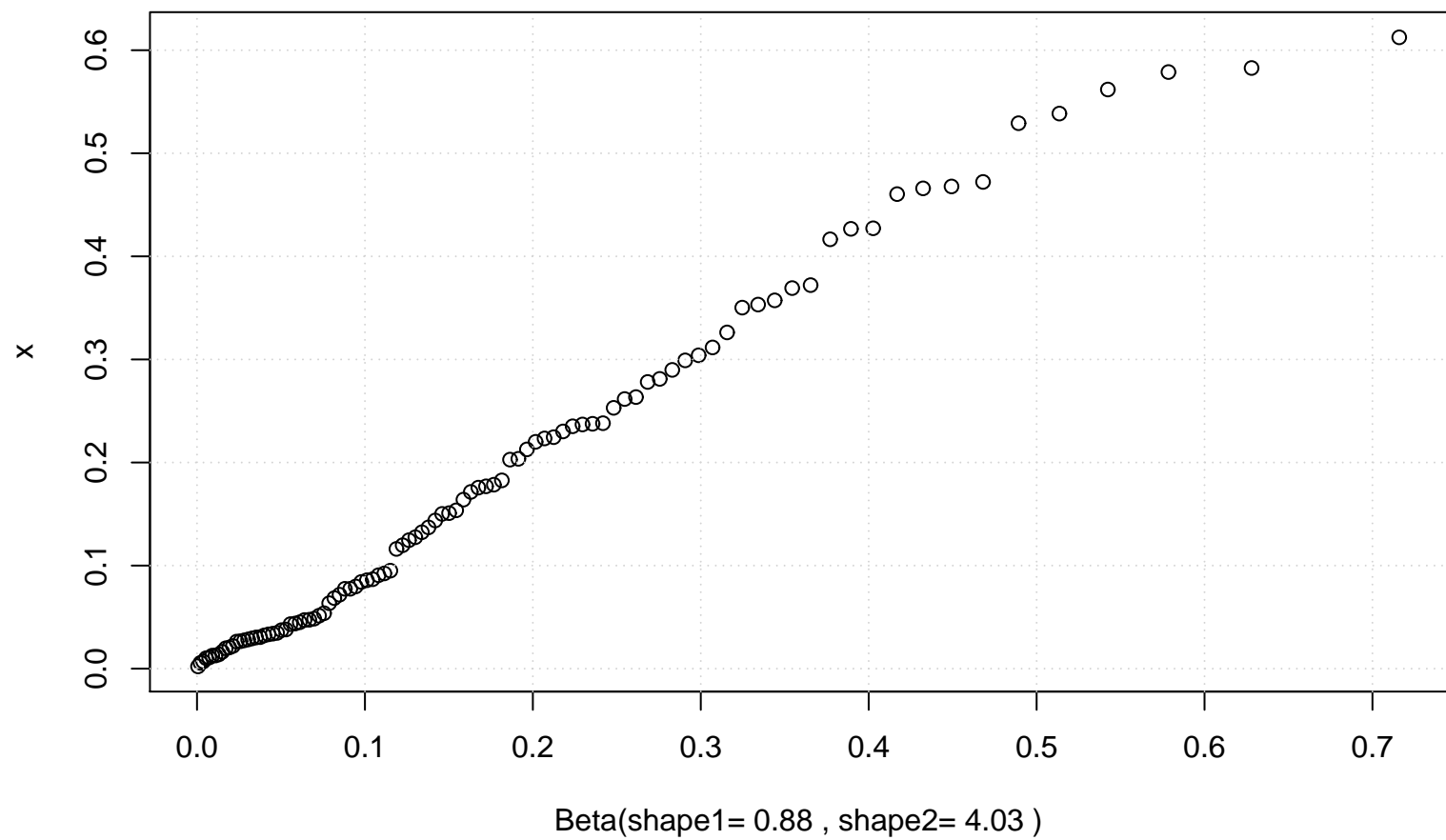
QQ plot (Beta)
