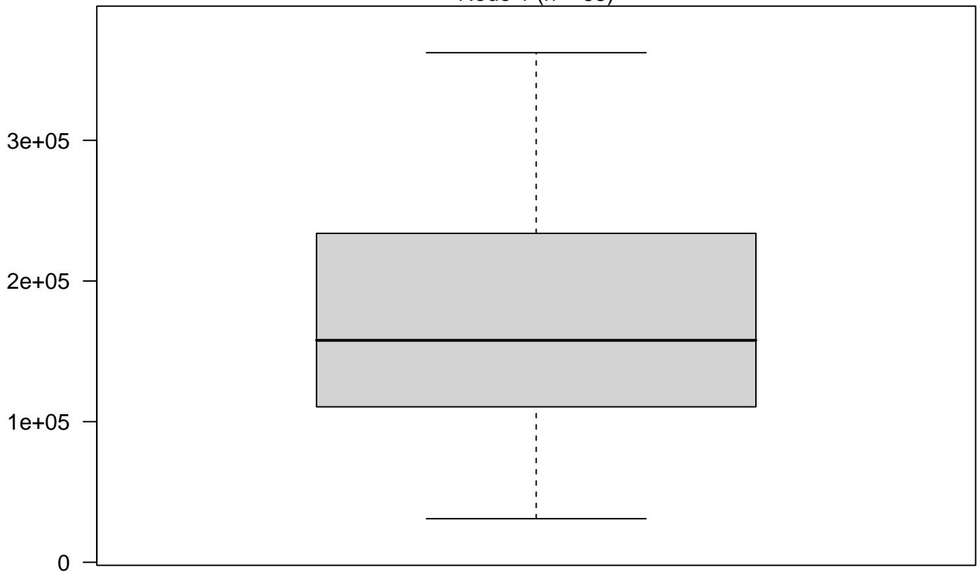
Node 1 (n = 68)
