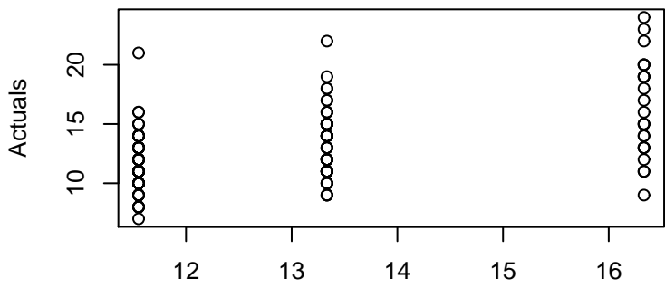
Actuals versus Predictions
