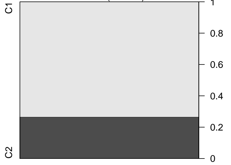
Node 3 (n = 132)
