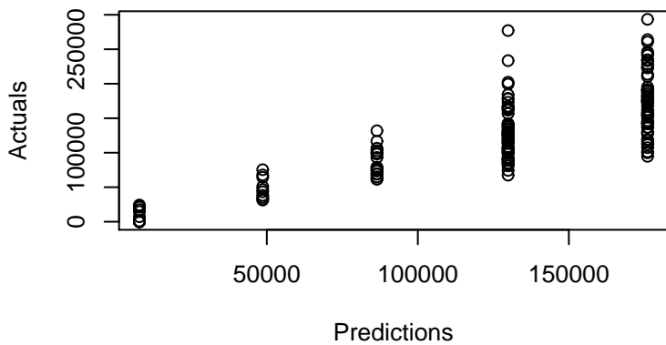
Actuals versus Predictions
