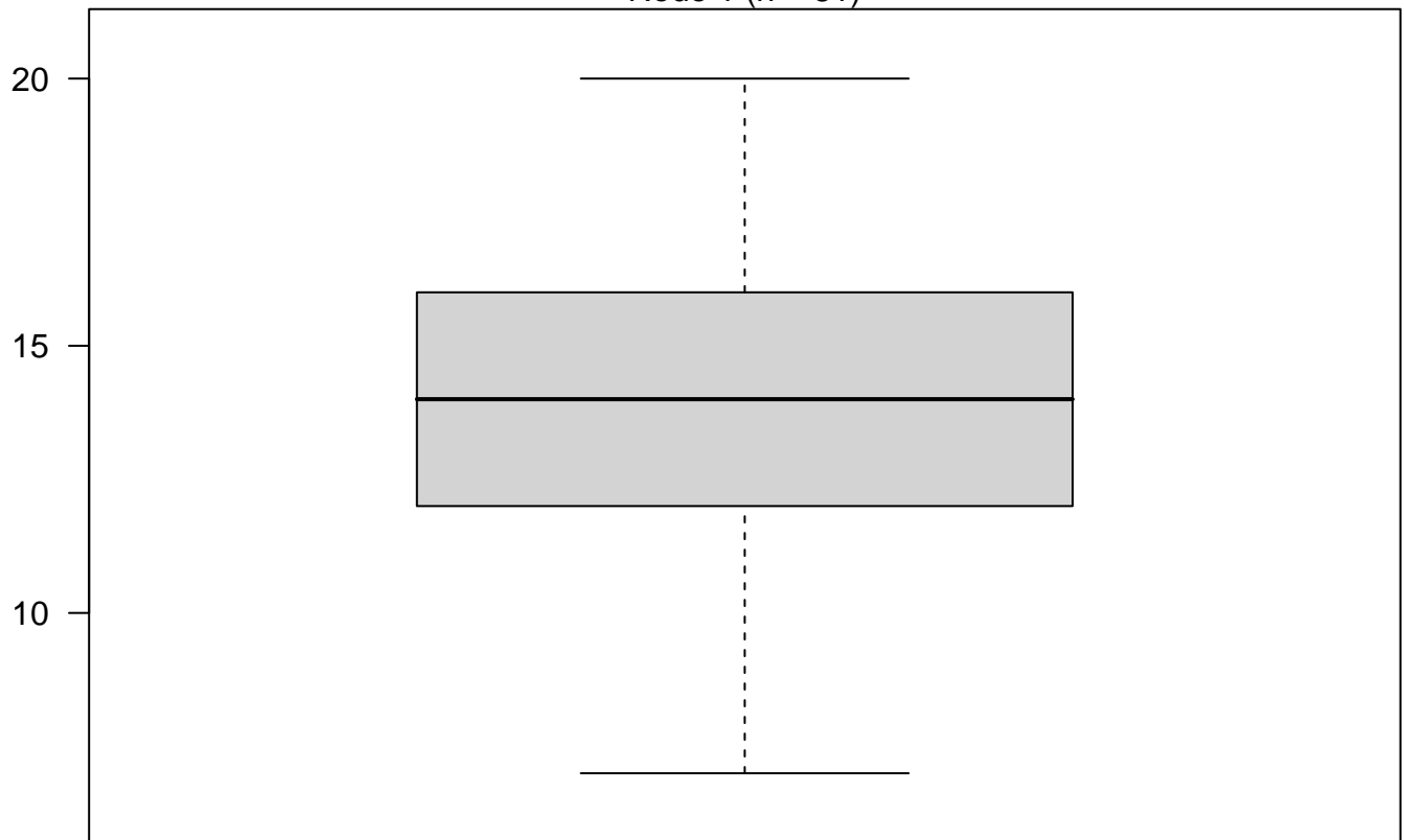
Node 1 (n = 81)
