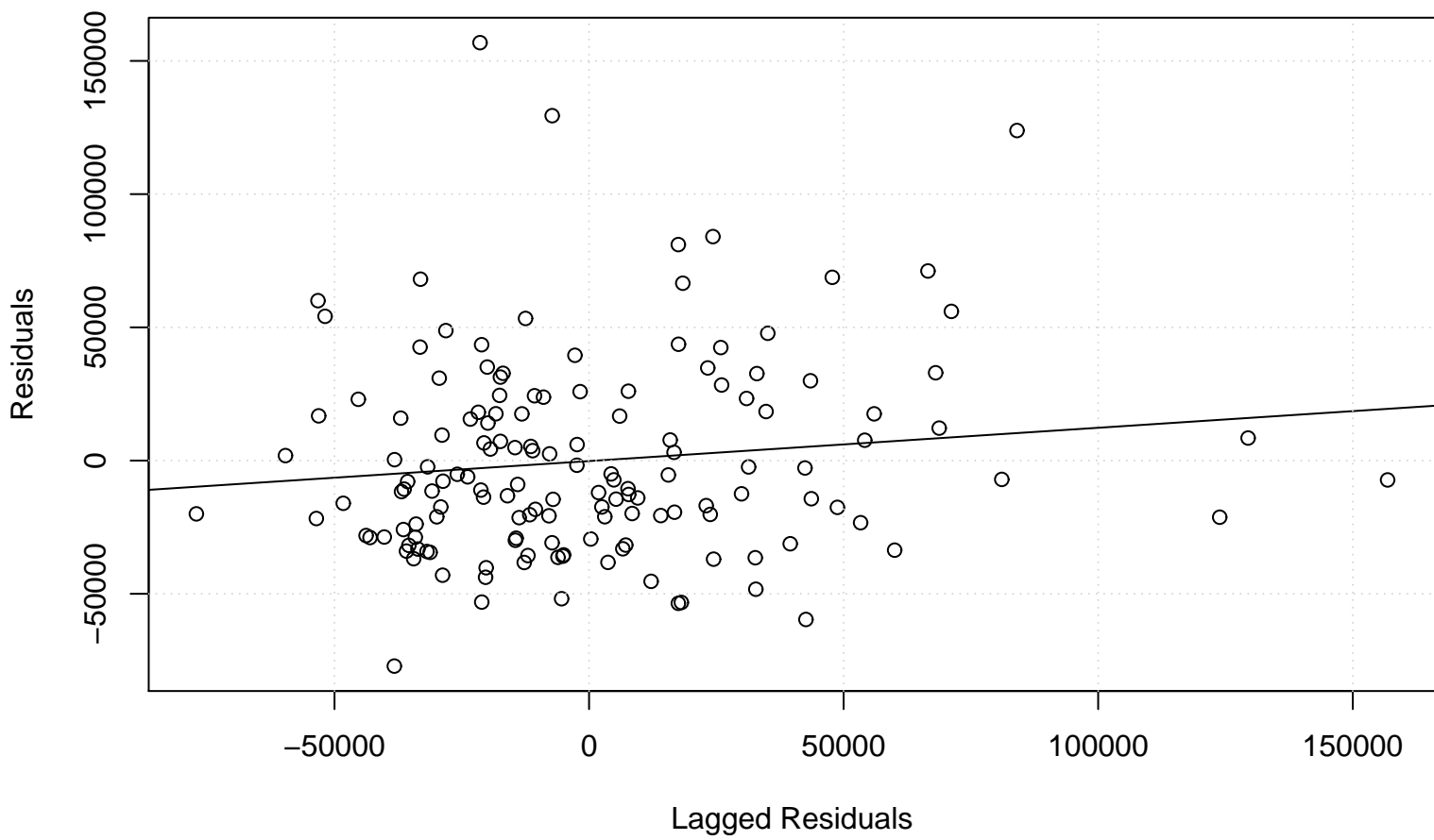
Lag plot
