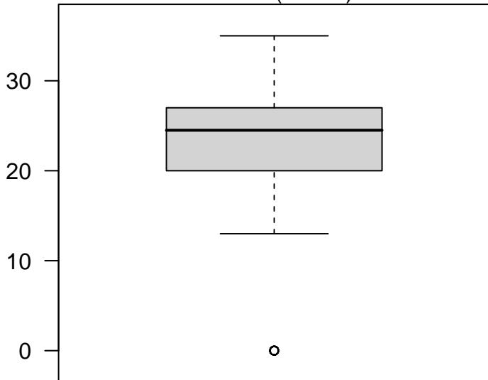
Node 2 (n = 62)
