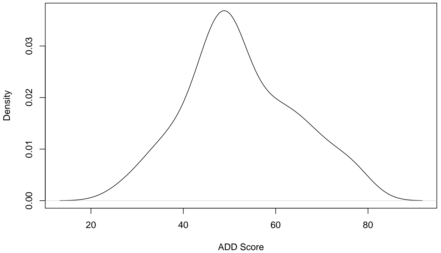
density.default(x = x)
