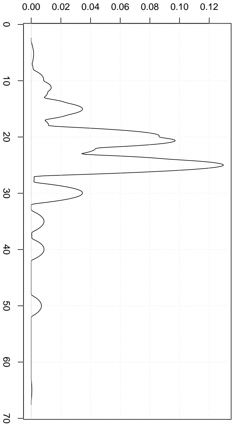
Epanechnikov Kernel
