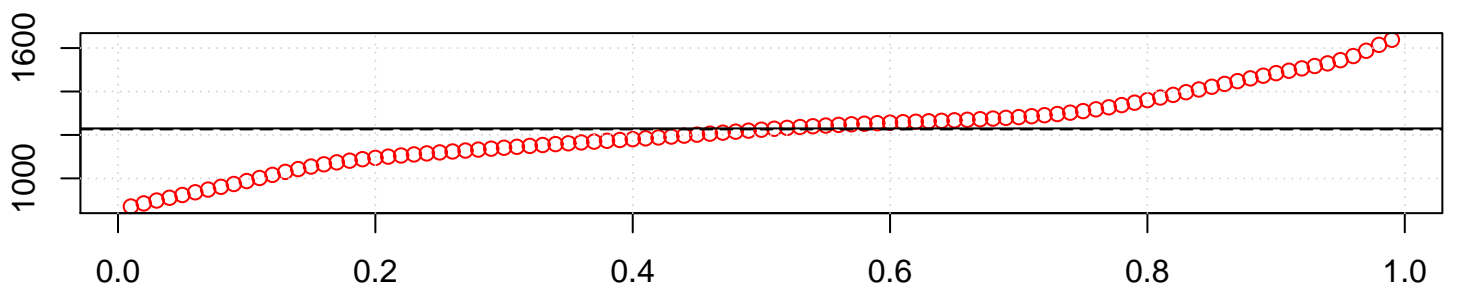
Harrell–Davis Quantiles
