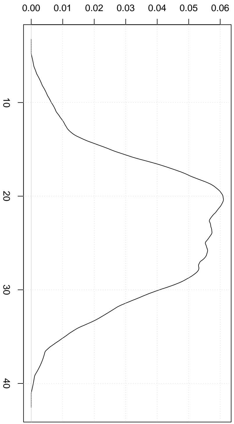
Epanechnikov Kernel
