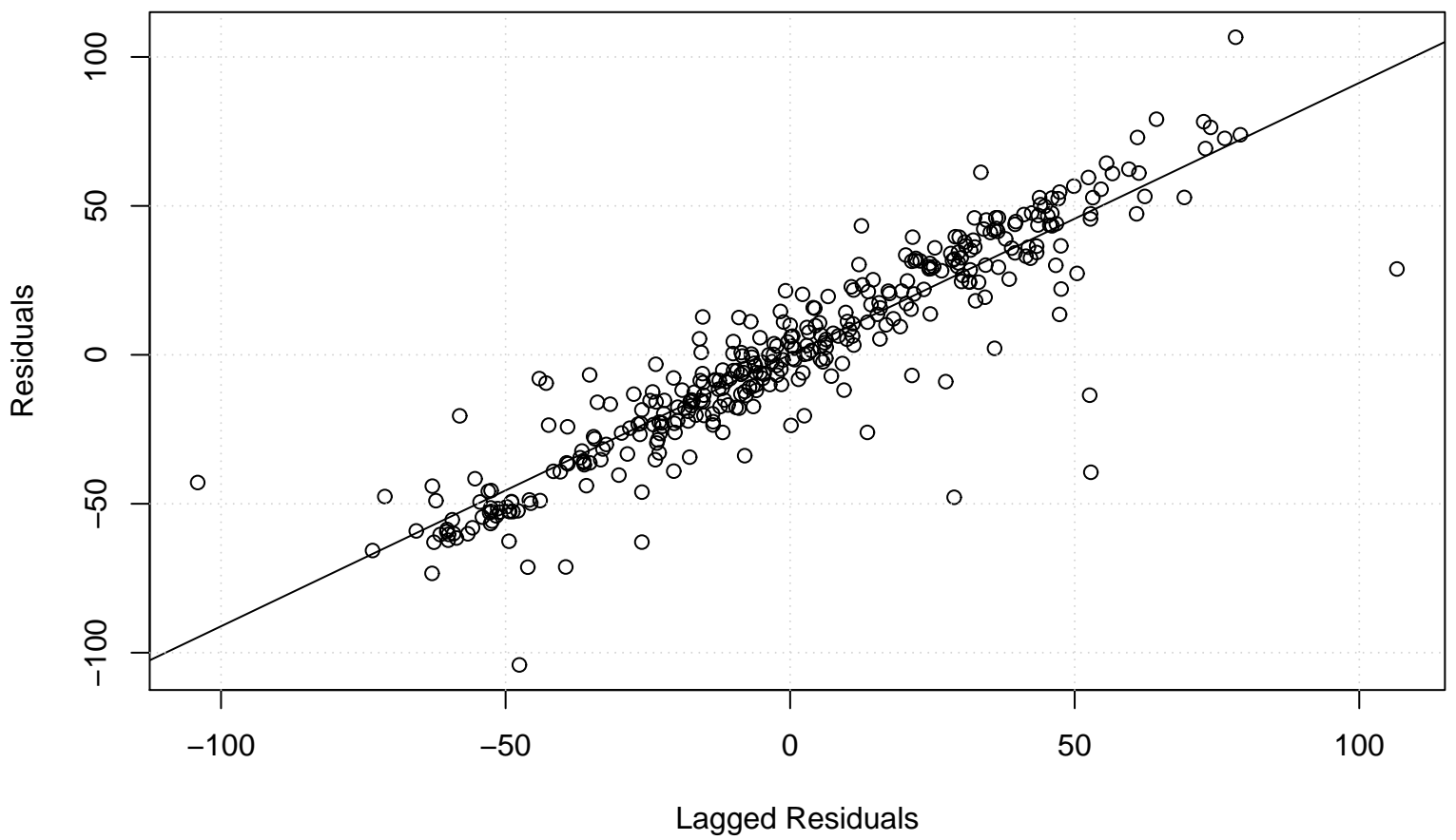
Lag plot
