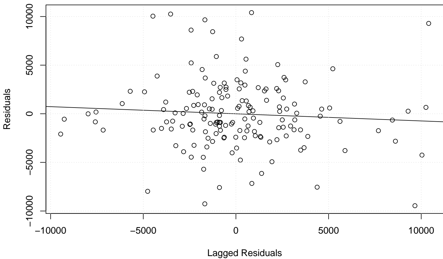
Lag plot
