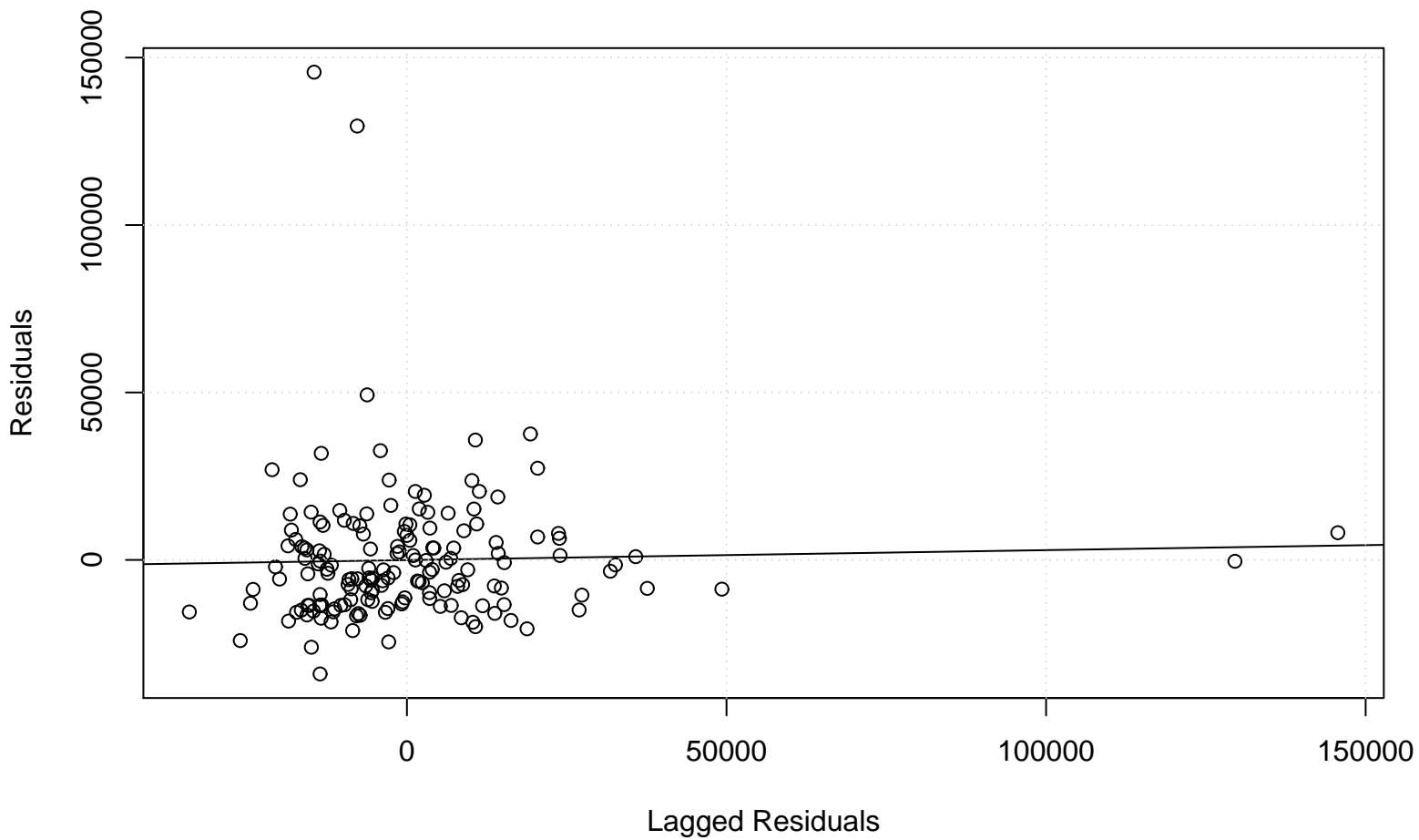
Lag plot
