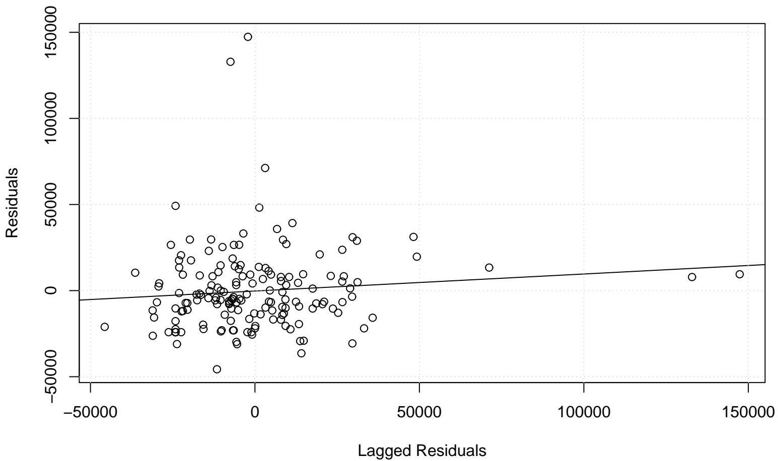
Lag plot
