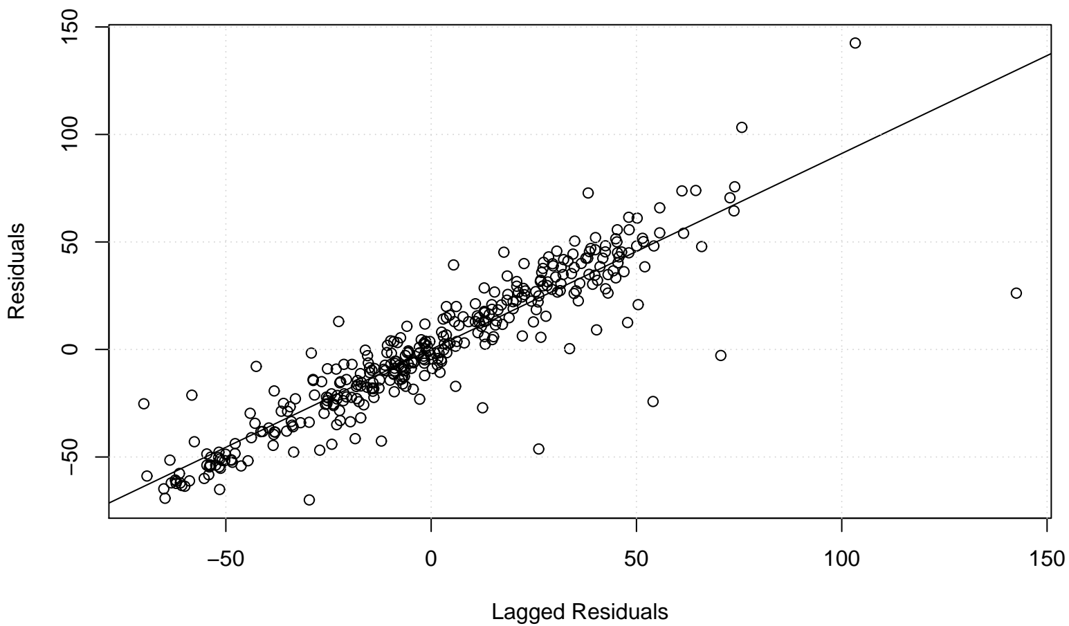
Lag plot
