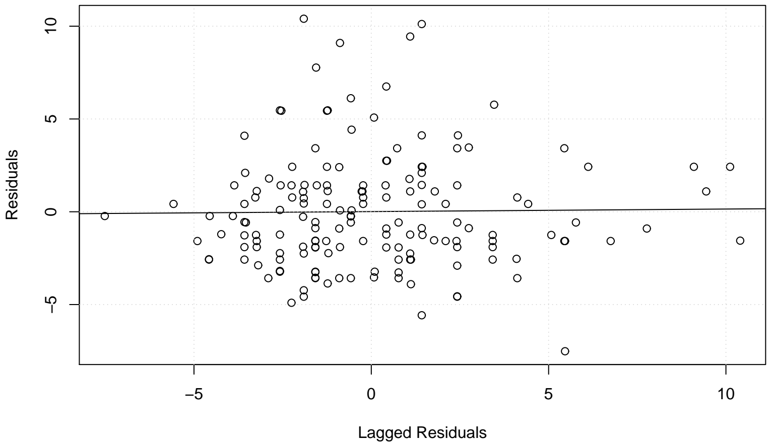
Lag plot
