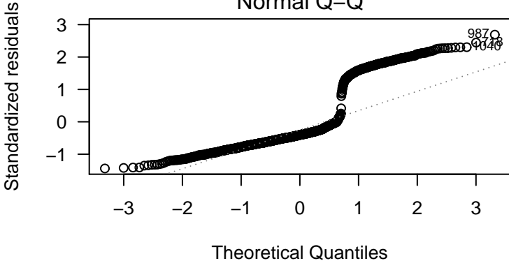
Normal Q-Q
