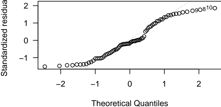
Normal Q-Q
