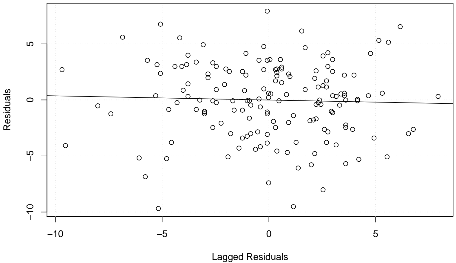
Lag plot
