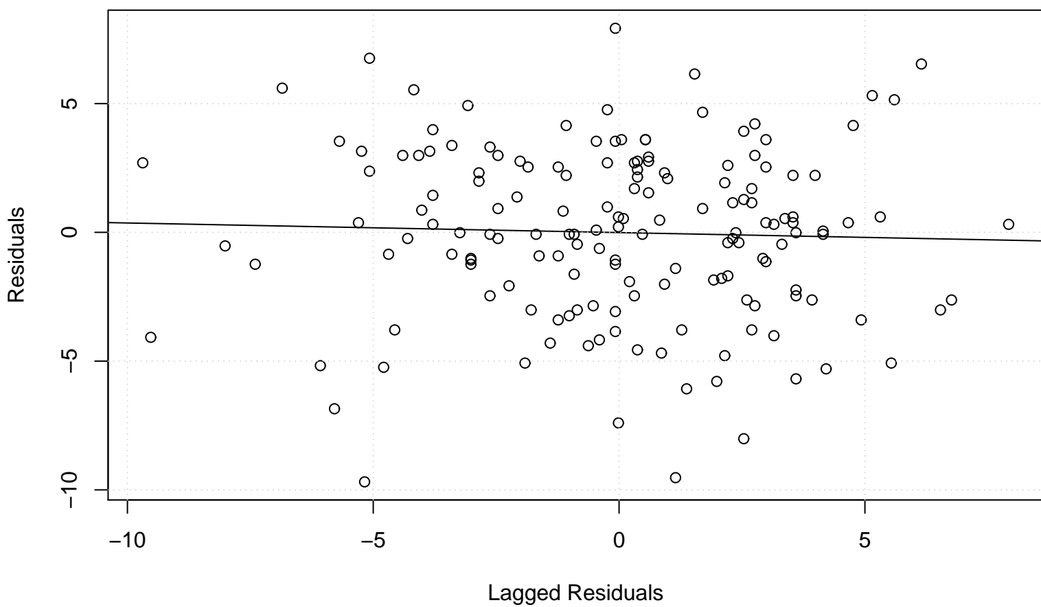
Lag plot
