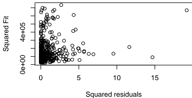
Sq.Resid vs. Sq.Fit
