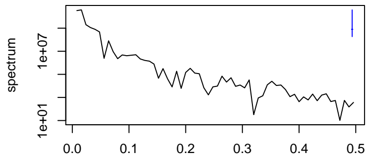
Trend
