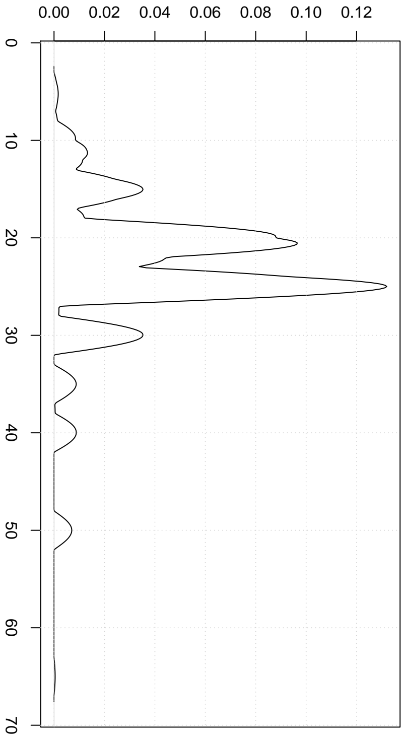
Optcosine Kernel
