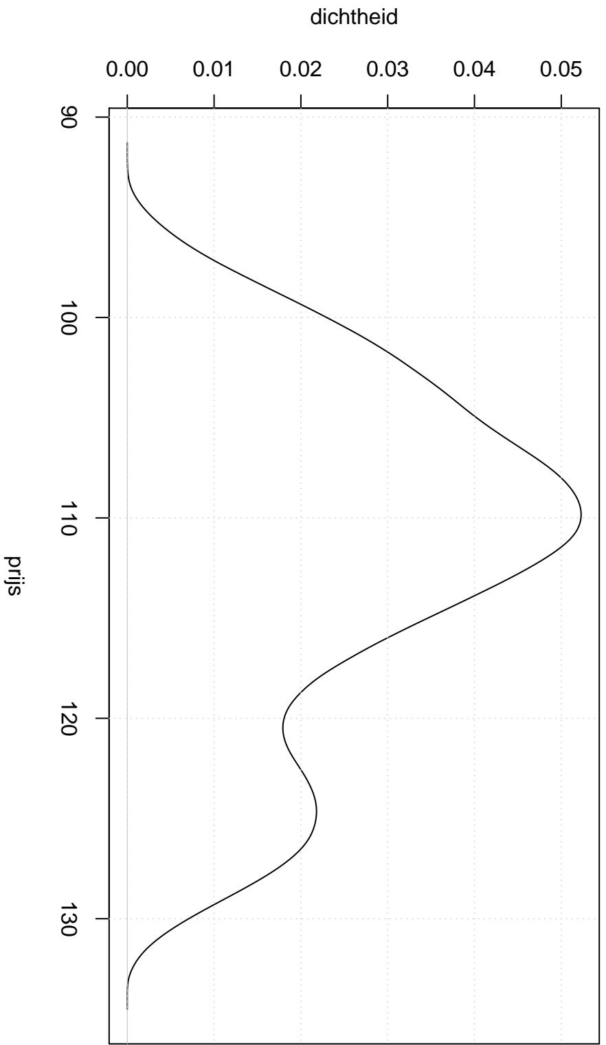
Cosine Kernel
