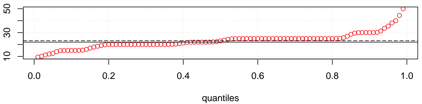
Harrell–Davis Quantiles
