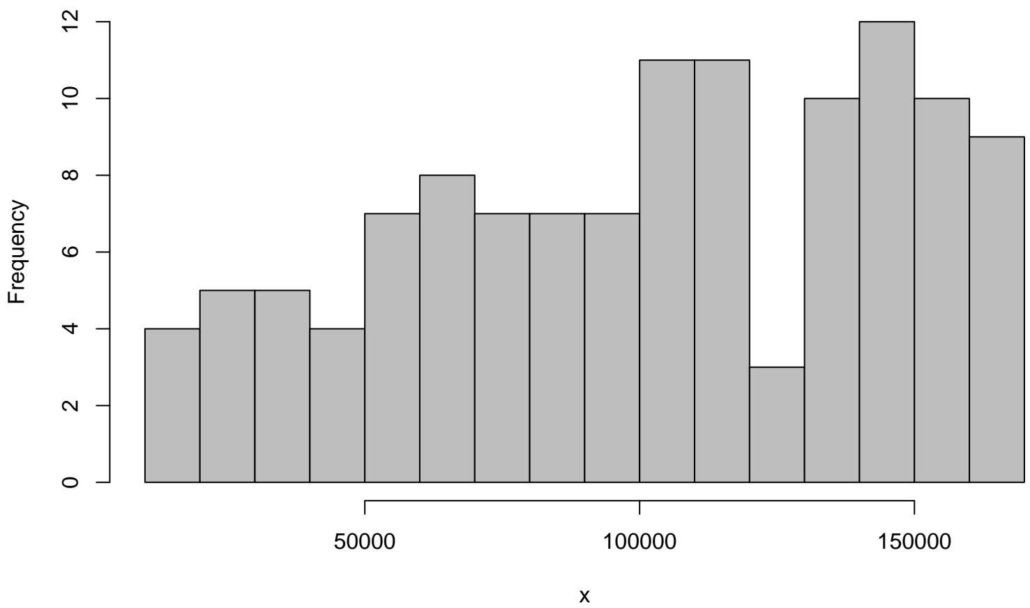
Histogram: 15 klassen
