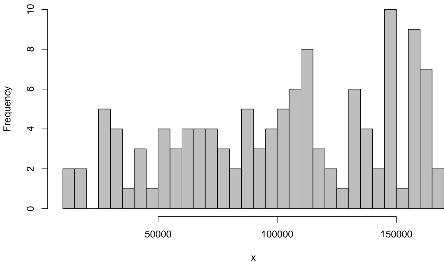
Histogram: 25 klassen
