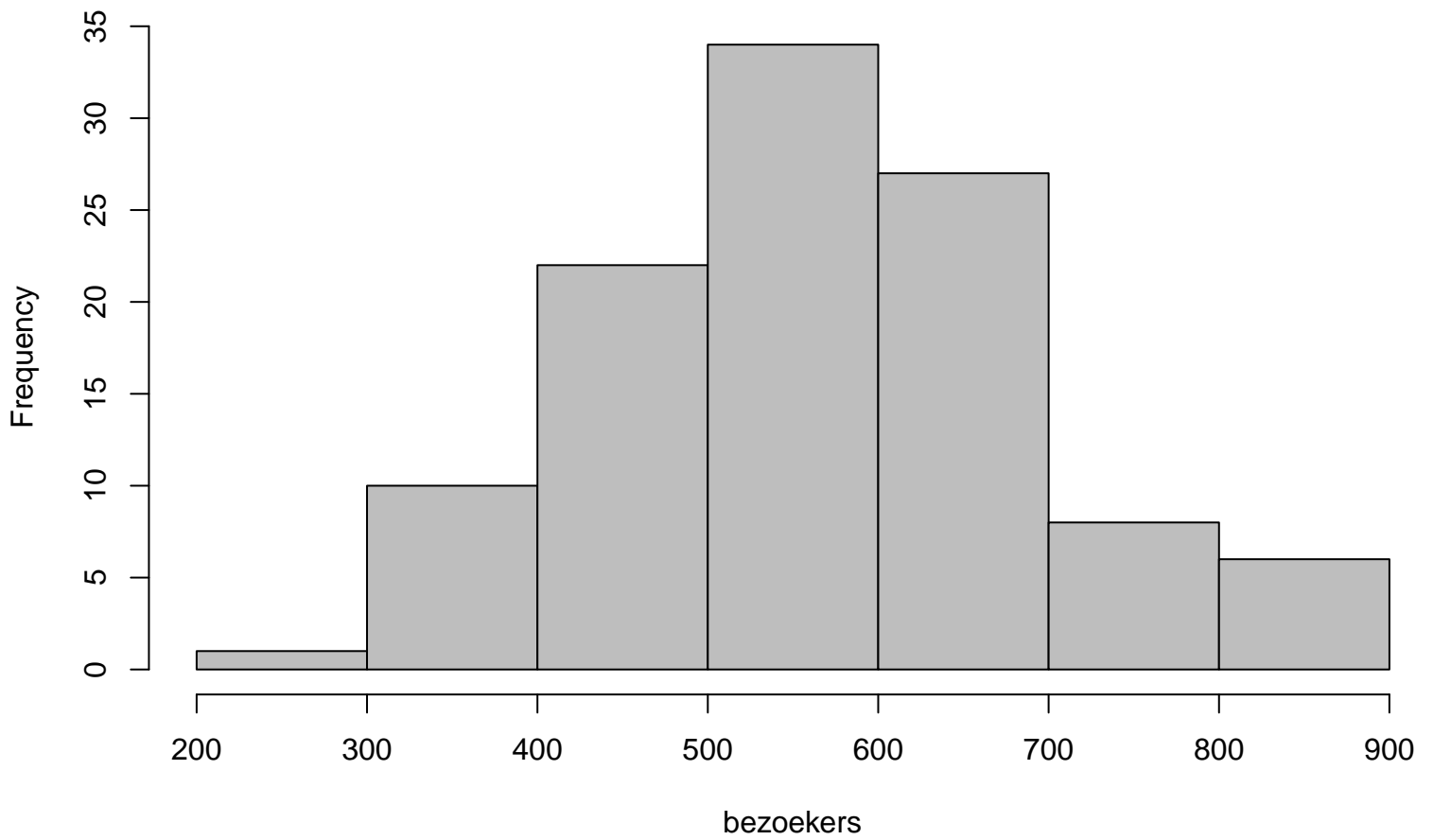
Histogram bezoekers
