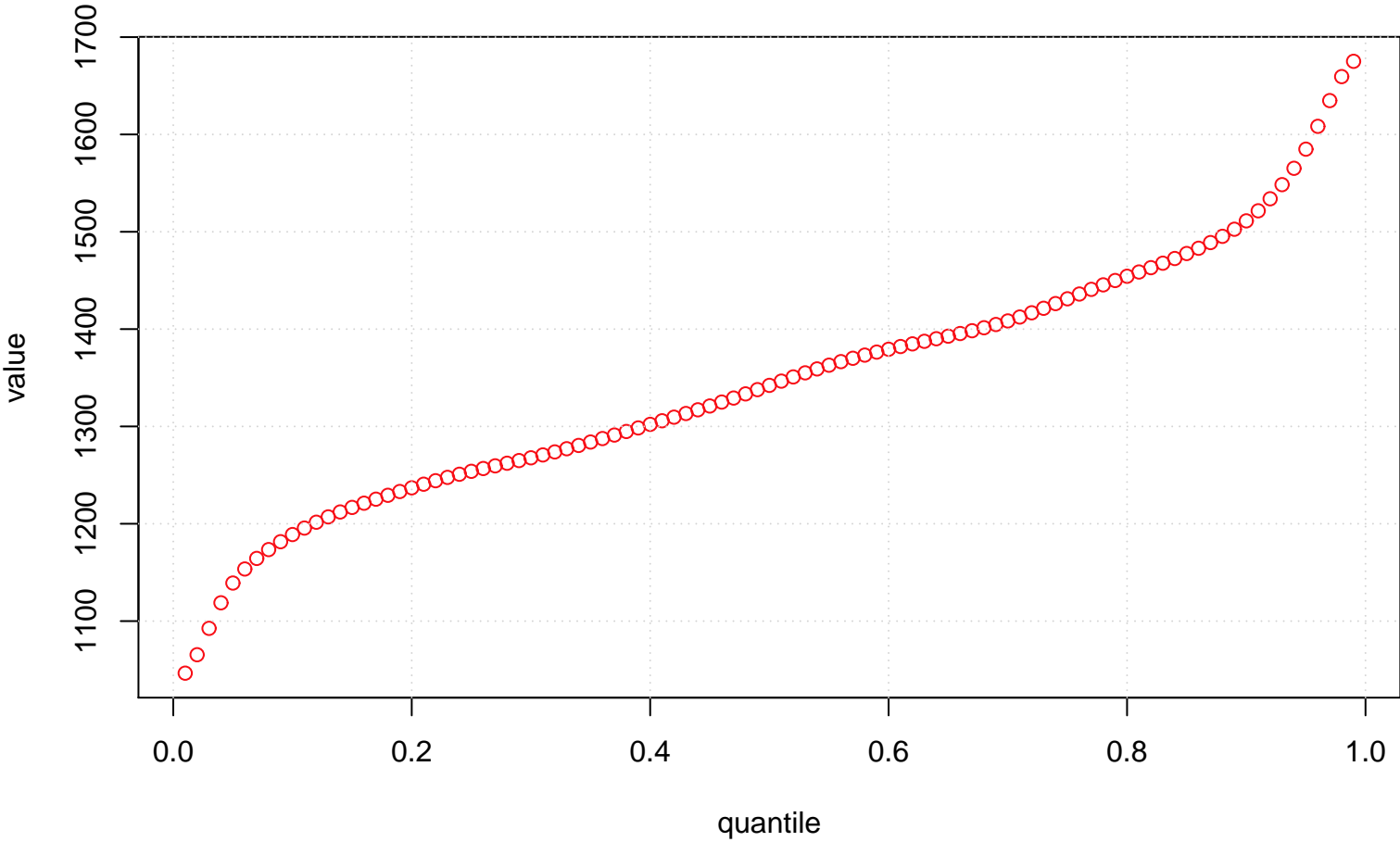
HD Quantiles Aantal bezoekers MOMA
