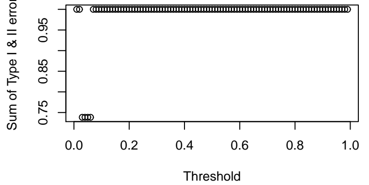
(1-Sens.) + (1-Spec.)
