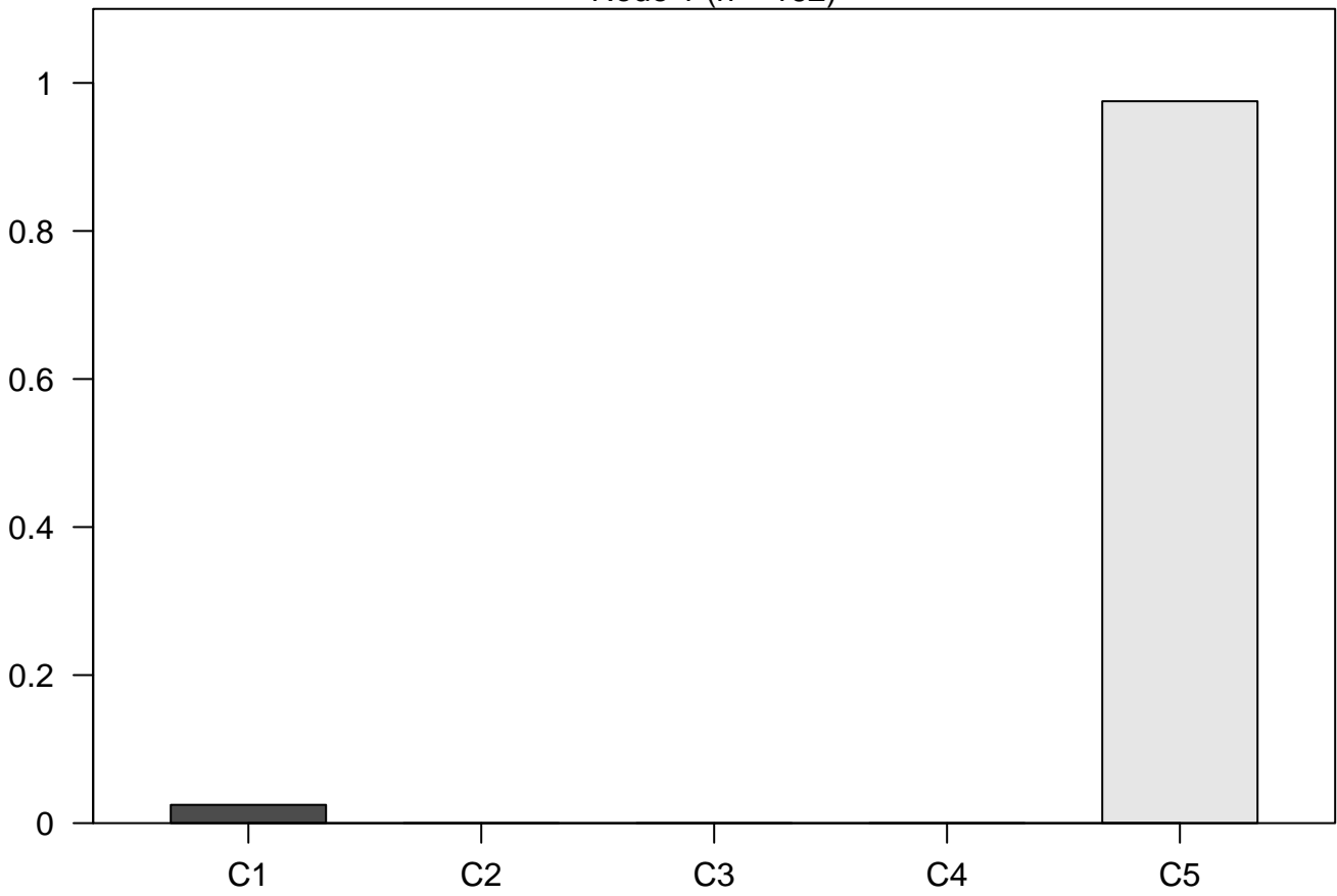
Node 1 (n = 162)
