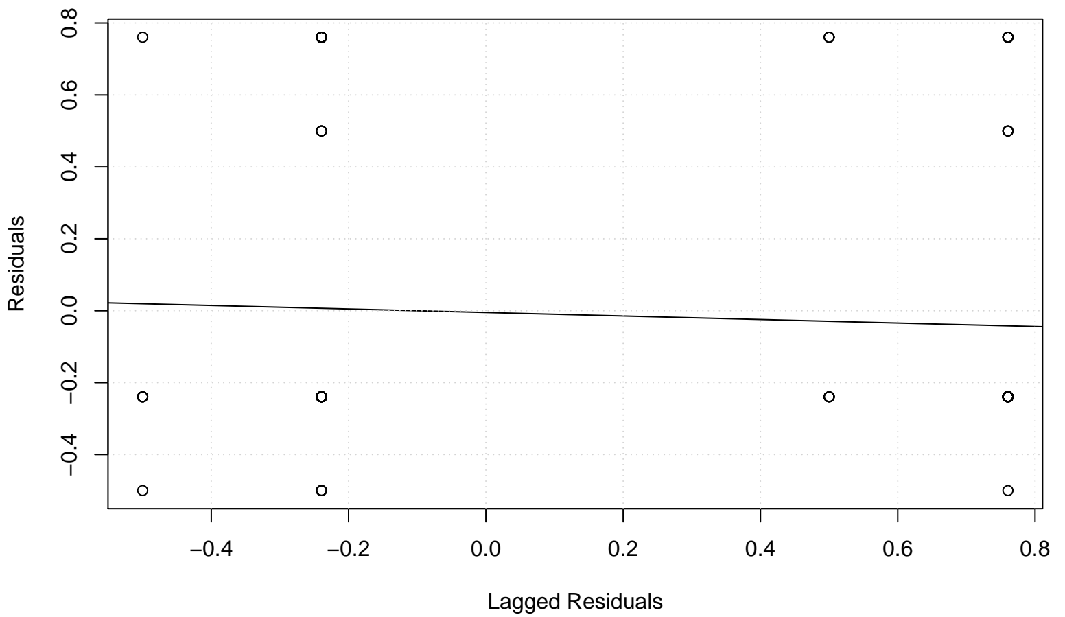
Lag plot
