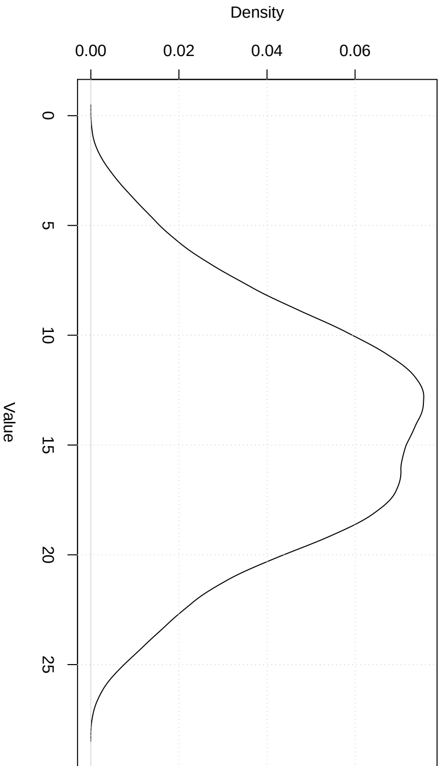
Cosine Kernel
