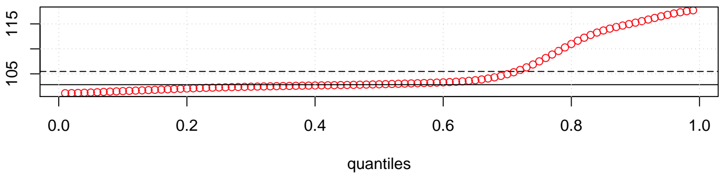
Harrell–Davis Quantiles
