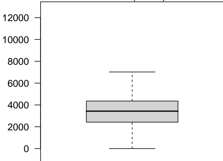
Node 2 (n = 28)
