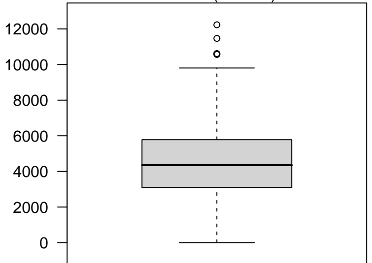
Node 3 (n = 192)
