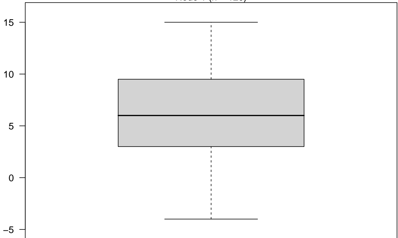
Node 1 (n = 120)
